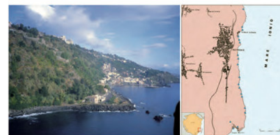
Fig. 1 - Le manifestazioni di acque sotterranee lungo il litorale di Acireale
