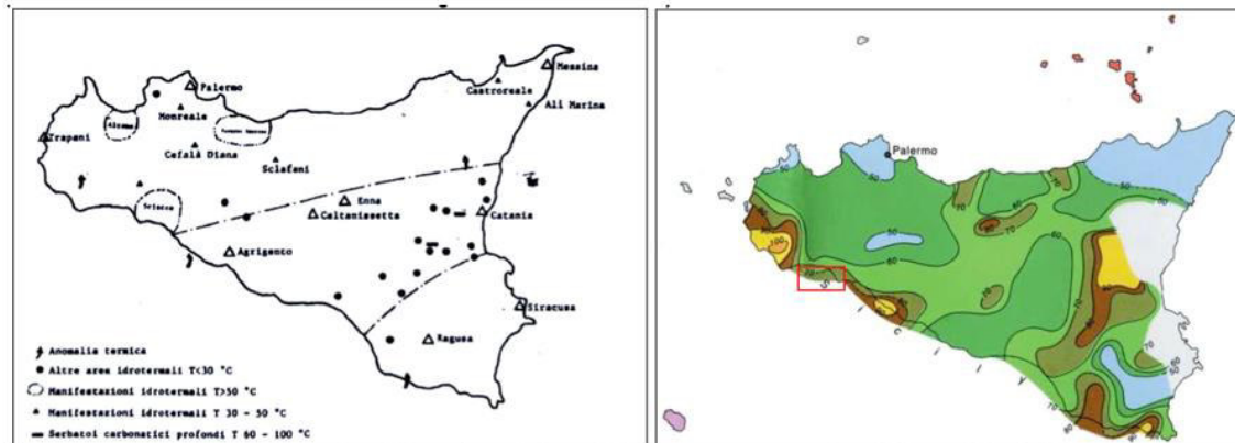
Fig. 96: distribuzione delle manifestazioni termali siciliane e range geotermico a 2000 metri di profondità
