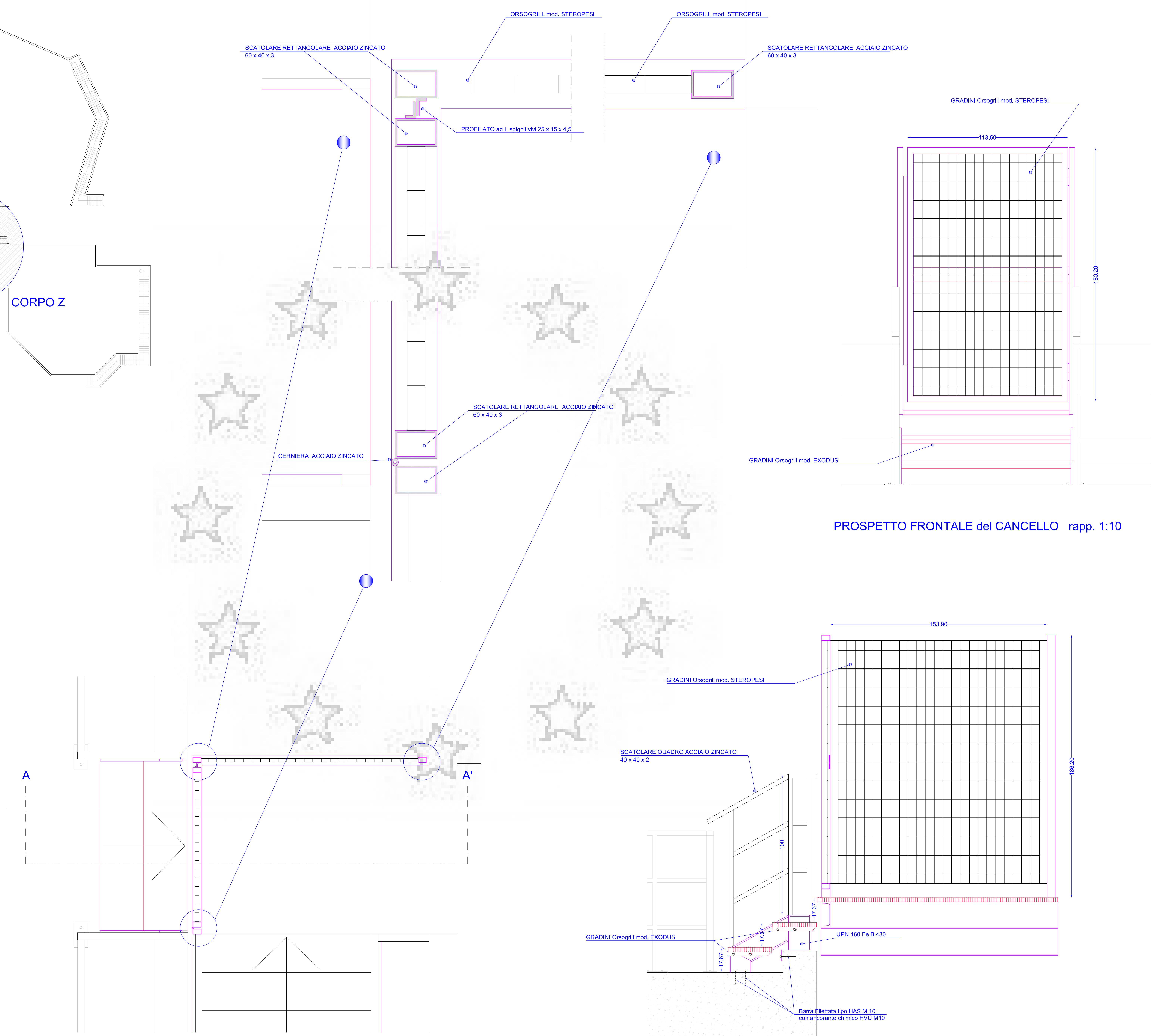
PIANTA CANCELLO E RINGHIERA TRA I CORPI C e Z rapp. 1:10
