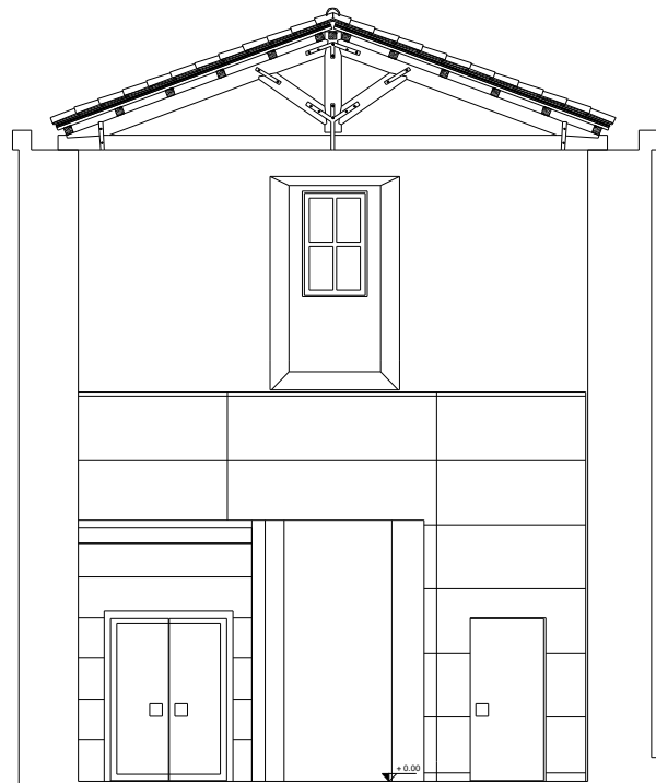
C - C'
