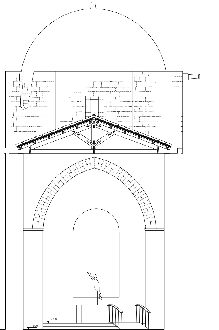
D - D'
