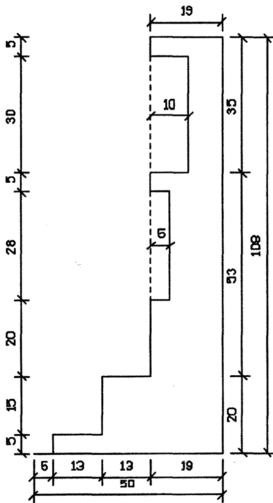
VISTA LATERALE BLOCCO CENTRALE
