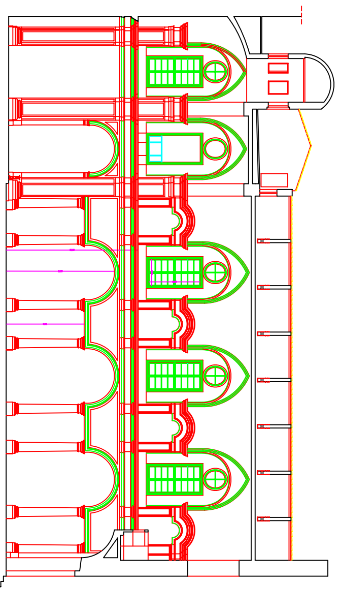
SEZIONE B-B
