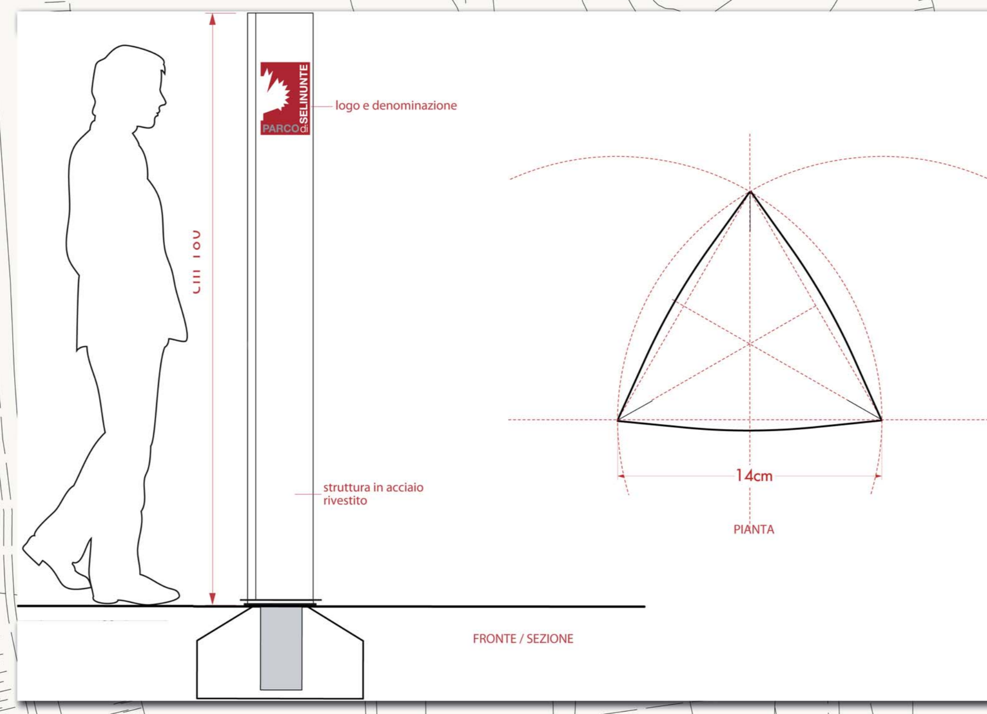
palina / totem - schema geometrico
