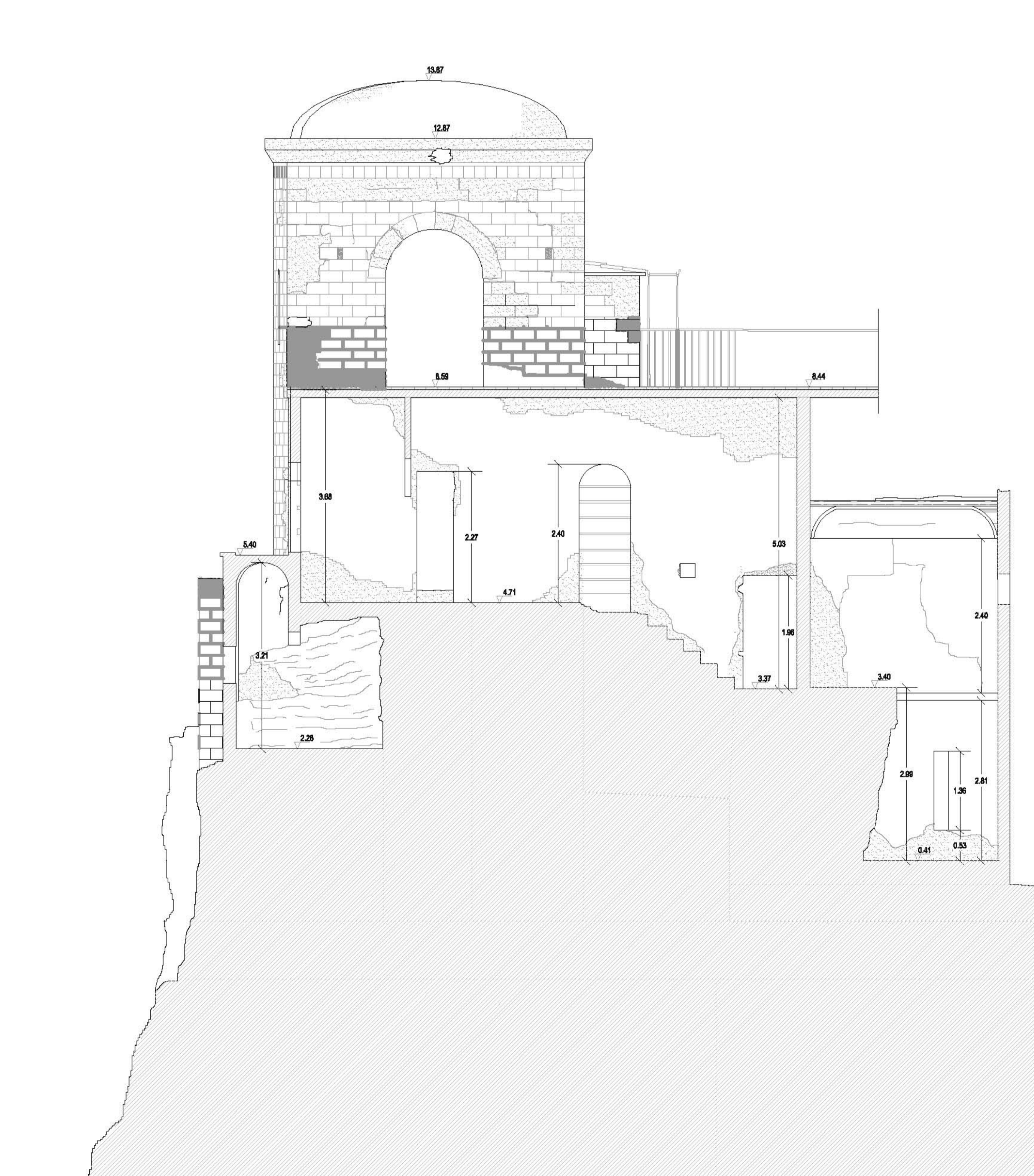
Sezione B-B
