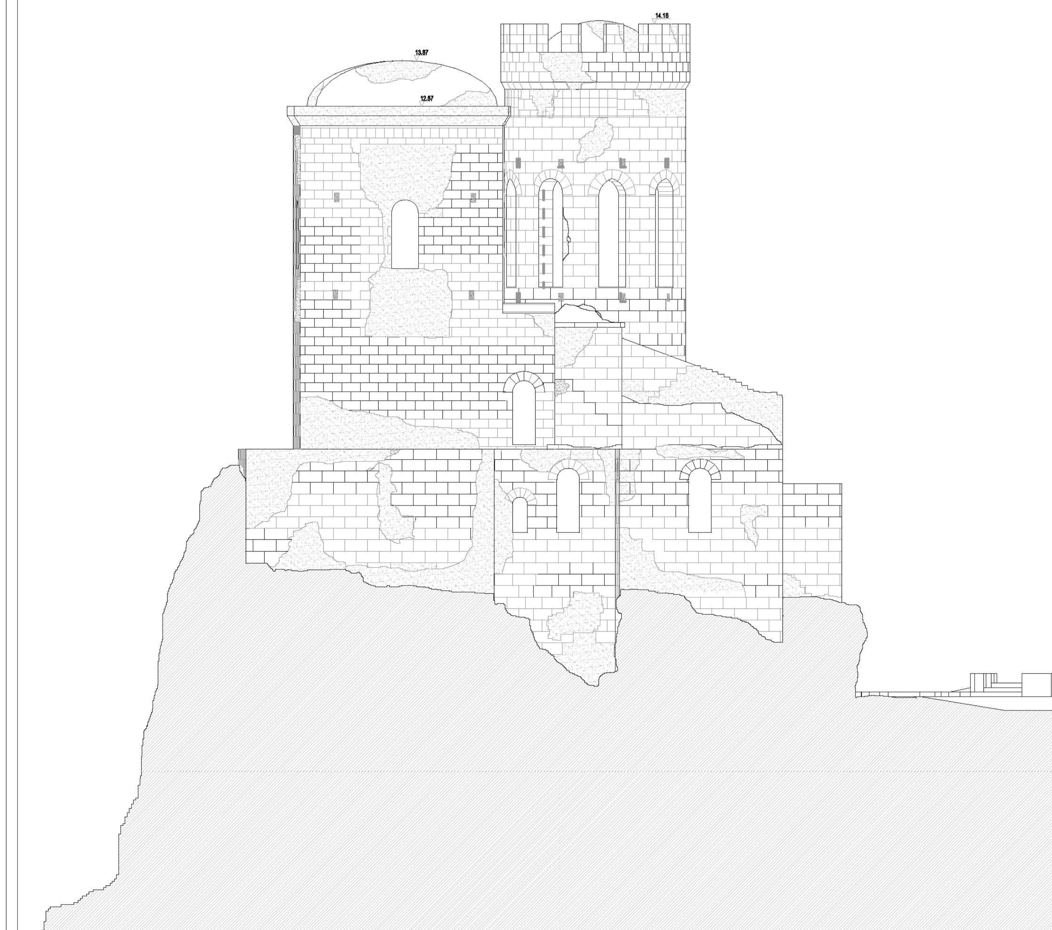
Prospetto Nord
