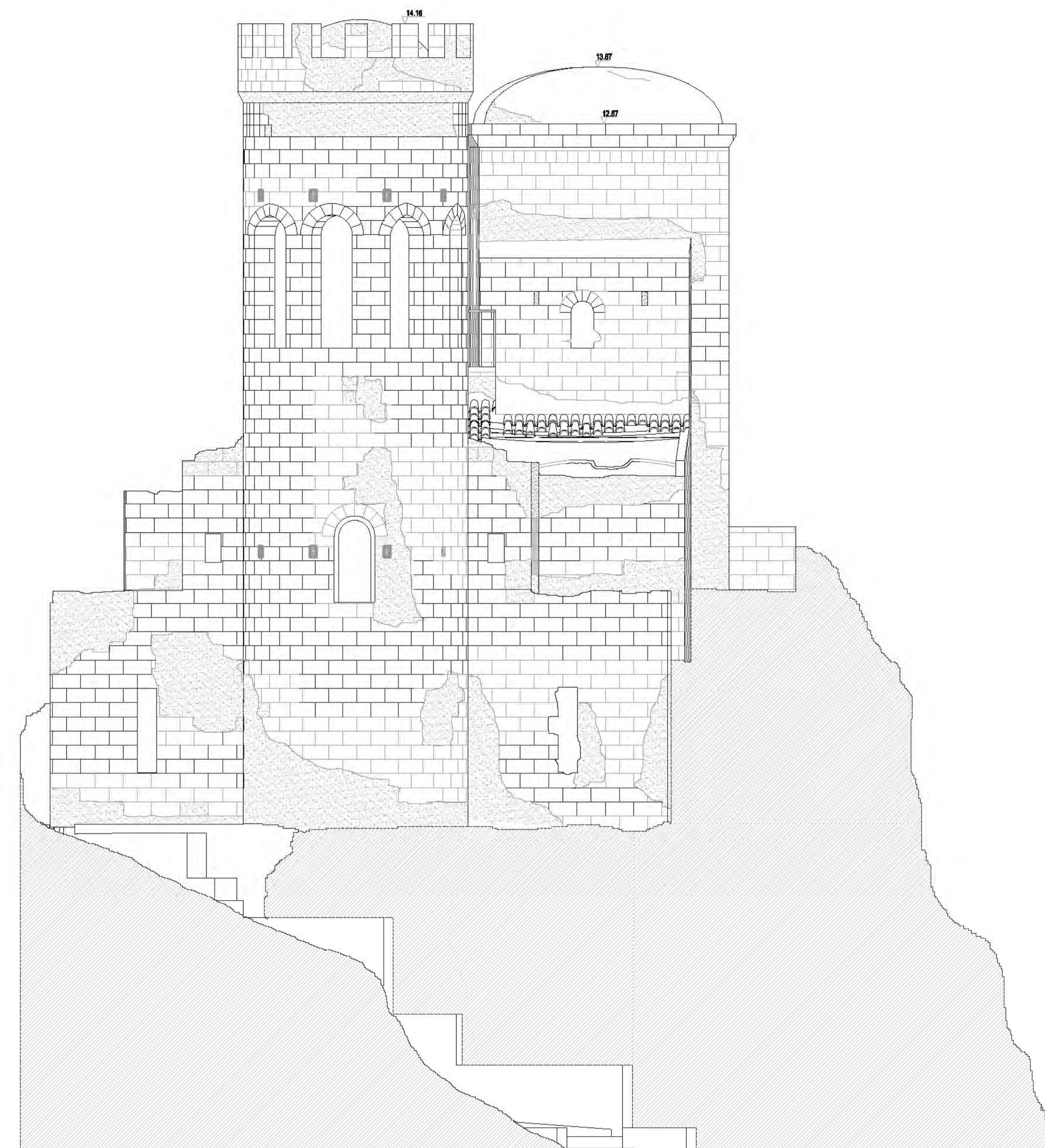
Prospetto Sud
