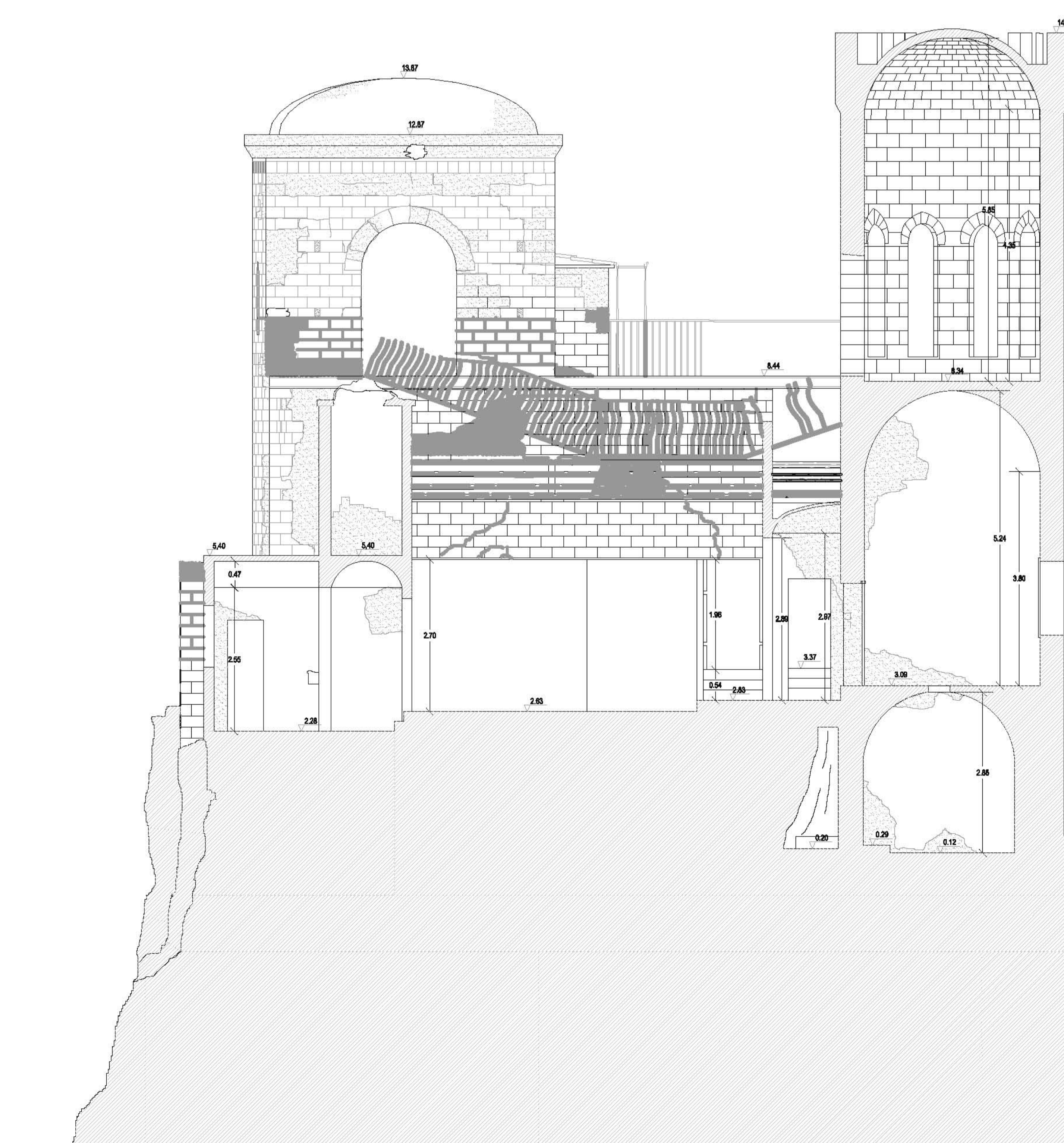
Sezione A-A
