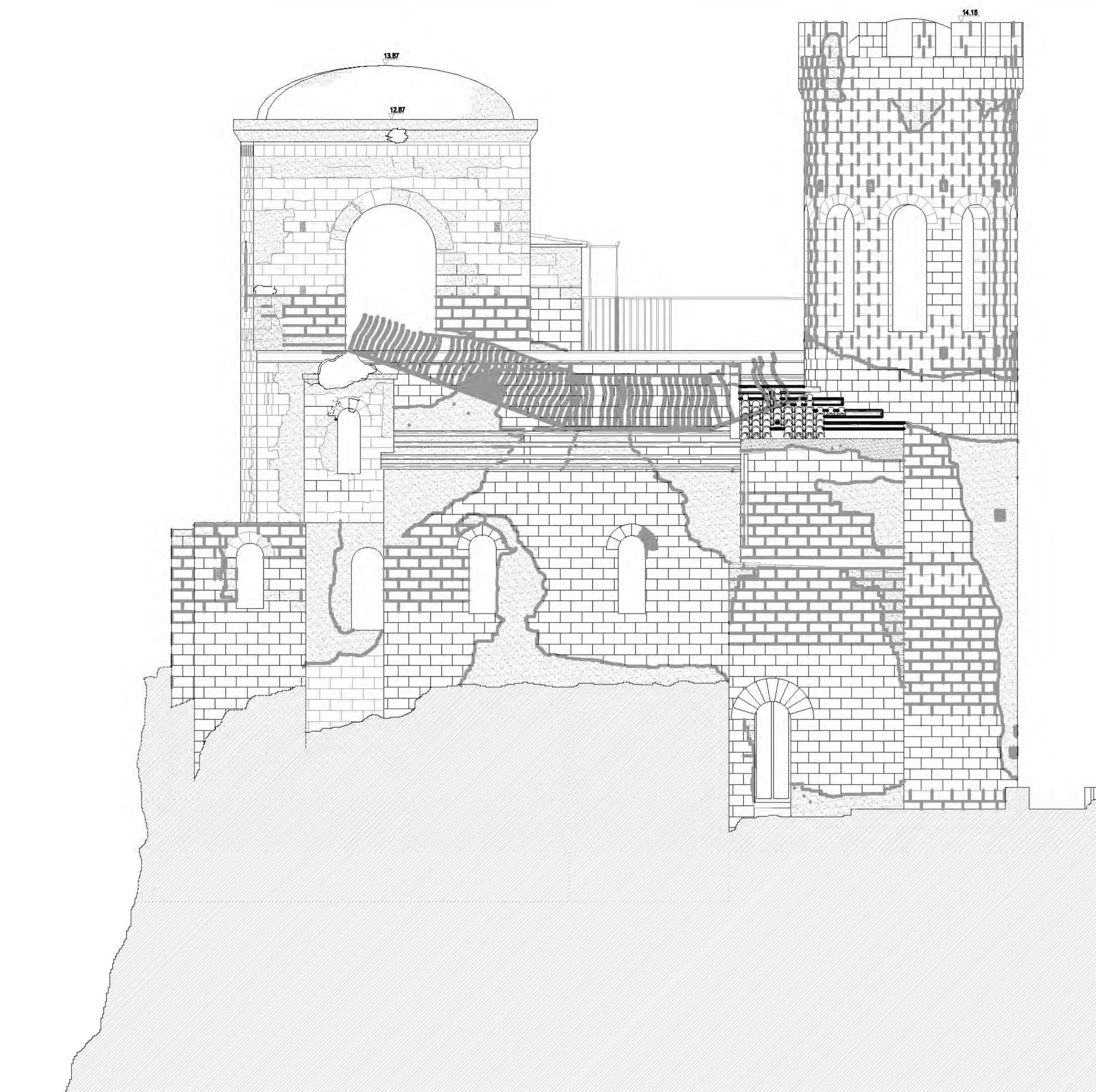
Prospetto Ovest
