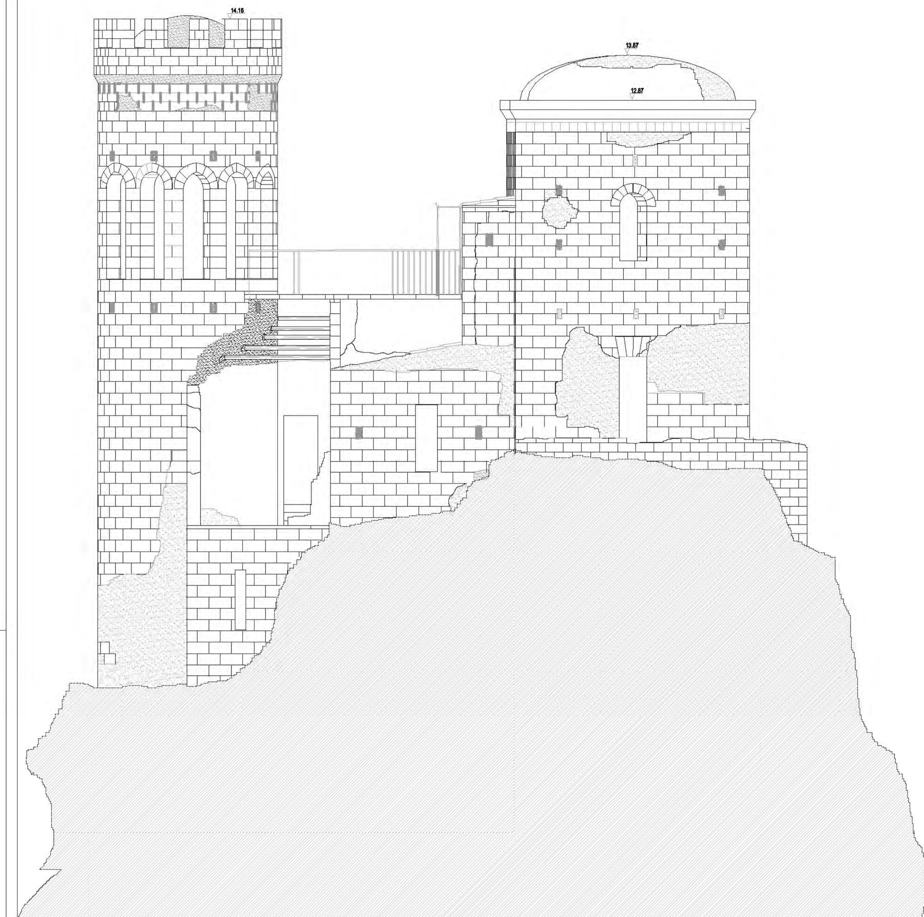
Prospetto Est
